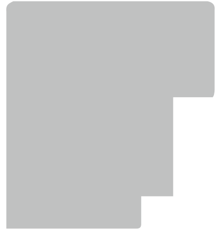
Bredde 55 mm - Høyde 60 mm Falsbredde 21 mm / høyde 36 mm
